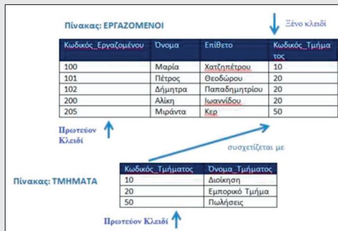
Σχήμα 3.5.6: Σχεσιακό μοντέλο
